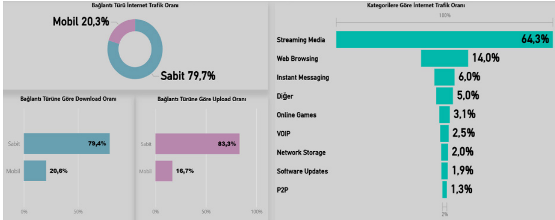
Şekil 3-12 Toplam Trafiğin Dağılımı
