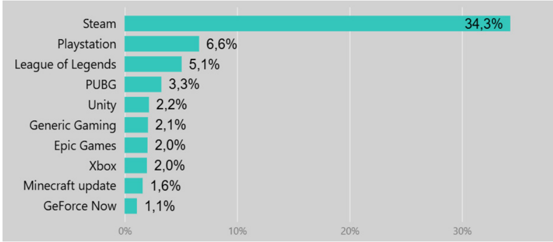
Şekil 3-18 Online Games Kategorisinde Kullanılmakta Olan Uygulamalar
